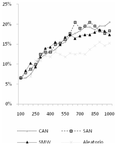
Fig. 1. Top candidato
