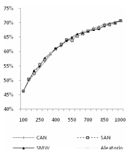
Fig. 4. Recall 20
