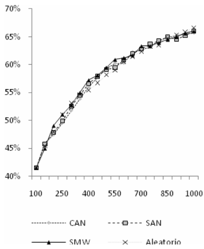
Fig. 3. Recall 15
