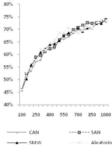
Fig. 2. Top 10
