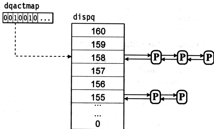
SVR4 dispatch queues.
