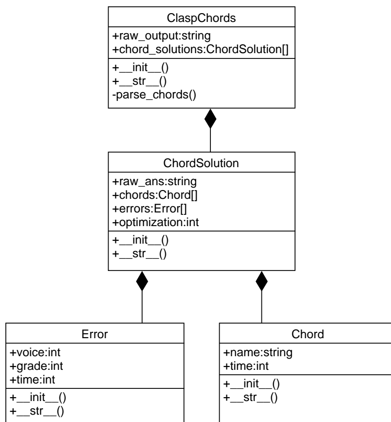
Figura A.5: Diagrama de clases de almacenamiento del módulo de armonización de la iteración 8
